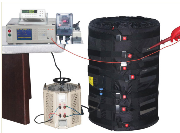
在热条件下总电流泄漏的测量设备
